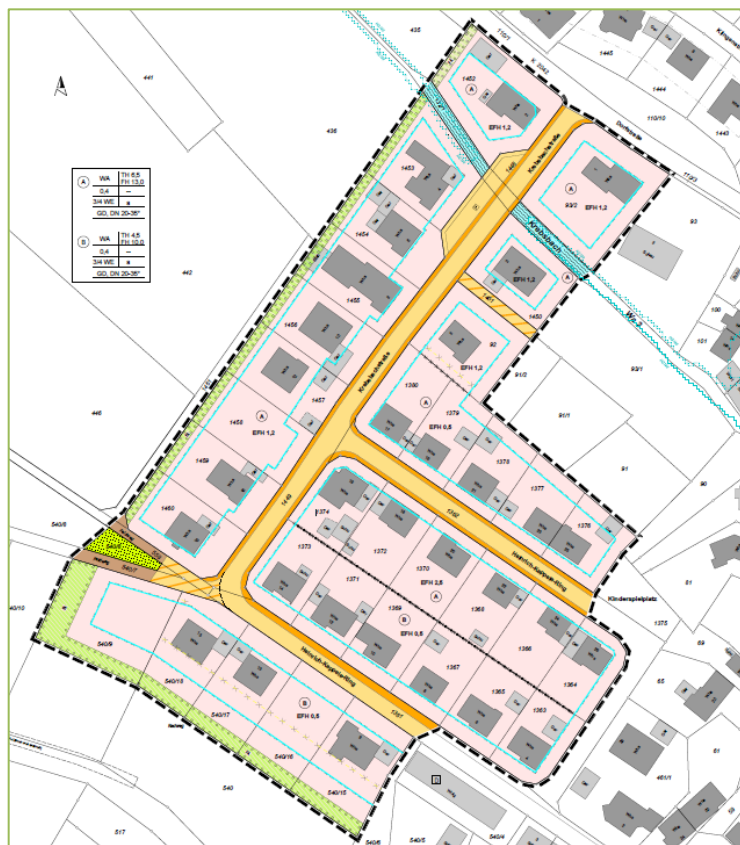
Abb.: Zeichnerischer Teil des neuen Bebauungsplans Brunnenberg / Gumpäcker Süd (unmaßstäblich)
