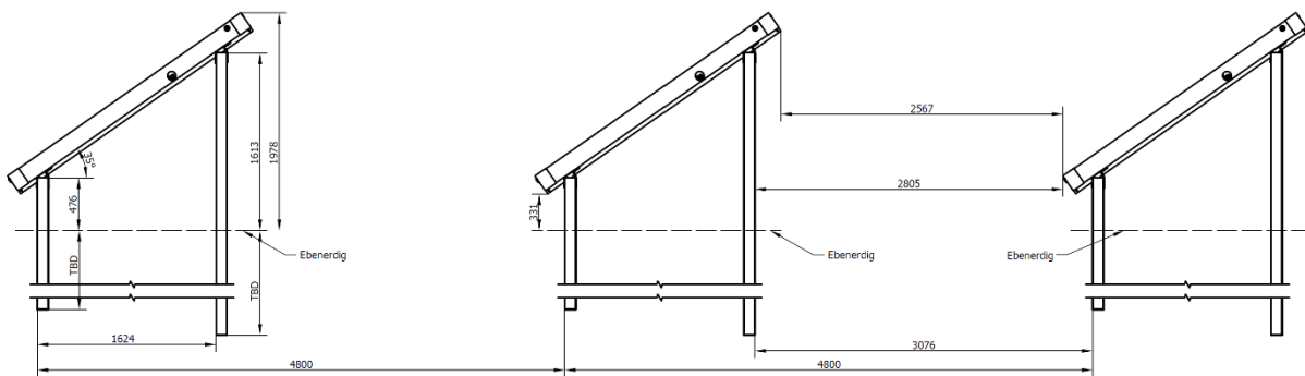
Abbildung 2 - Ostansicht Solaranlage mit Freiflächenmontagesystem
