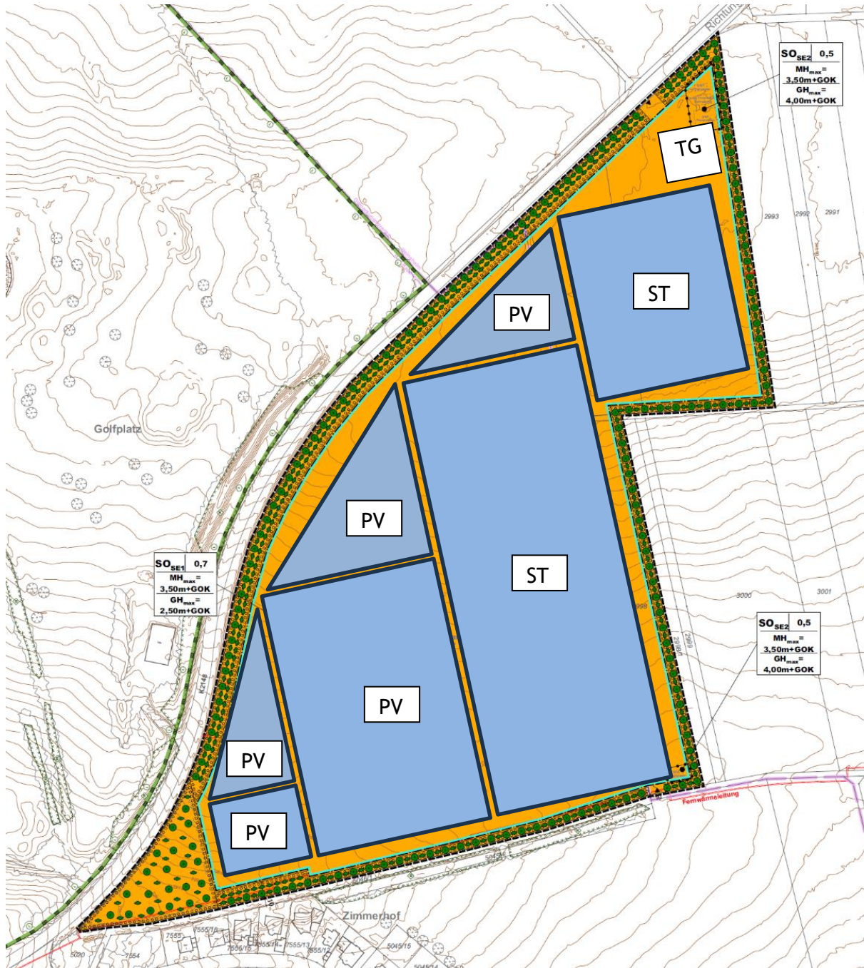
Abbildung 1 - Lageplan zu "Solaranlage Kiesgrubenäcker"
